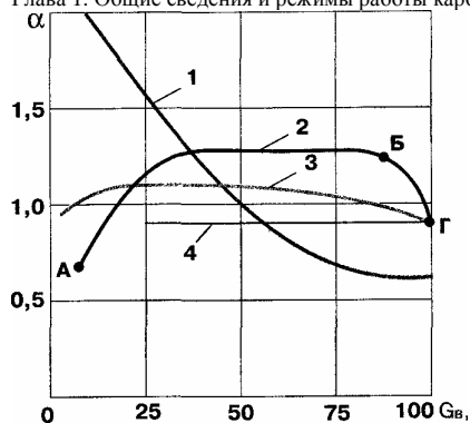
Рис. 1. Изменение \alpha при различных режимах работы двигателя: 1 - простейший карбюратор, 2 - идеальный карбюратор, 3 - нагрузочная характеристика, 4 - внешняя скоростная характеристика
