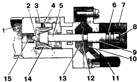
Рис. 28. Схема размещения регулировочного винта количества горючей смеси и ограничительной втулки карбюратора «Озон» с ЭПХХ
