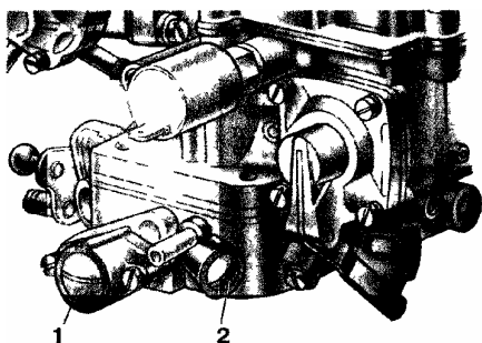
Рис. 25. Винты регулировки системы холостого хода: 1 - винт количества смеси; 2 - винт качества смеси
