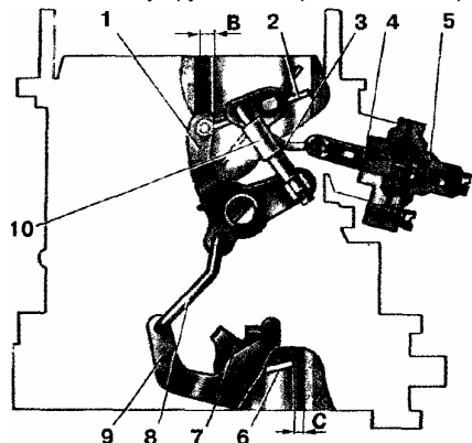
Рис. 23. Схема регуляции пускового устройства: 1 - рычаг привода воздушной заслонки, 2 - воздушная заслонка, 3 - тяга пускового устройства, 4 - рейка пускового устройства, 5 - регулировочный винт, 6 - дроссельная заслонка первичной камеры, 7, 9 - рычаги, 8 - тяга привода дроссельной заслонки, 10 - телескопическая тяга, В, С - пусковые зазоры заслонок
