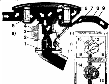
Рис. 14. Система вентиляции картера двигателя: I - при малой частоте вращения коленчатого вала двигателя, II - при большой частоте вращения коленчатого вала двигателя, а - схема системы вентиляции, б - работа золотникового устройства, 1 - впускной трубопровод, 2 - дроссельная заслонка, 3 - шланг отсоса картерных газов в задрроссельное пространство, 4 - карбюратор, 5 - фильтрующий элемент, 6 - воздушный фильтр, 7 - патрубок, 8 - пламегаситель, 9 - вытяжной шланг, 10 - золотниковое устройство, 11 - выходной канал, 12 - калиброванное отверстие, 13 - лыска оси, 14 - дополнительное отверстие 15 16 - нижняя и верхняя выемки
