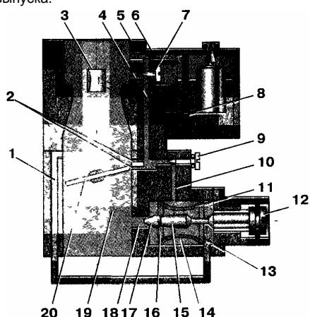
Рис. 5. Система АСХХ карбюратора типа «Озон»: 1 - обводной воздушный канал, 2 - переходные отверстия, 3 - диффузор, 4 - эмульсионный канал, 5 - воздушный жиклер, 6 - топливный жиклер АСХХ, 7 - подстроечный винт, 8 - топливный жиклер ГДС, 9 - винт качества, 10 - канал, 11 - кольцевой распылитель, 12 - винт количества, 13 - входная полость, 14 - топливные отверстия, 15 - конический стержень, 16 - выходная полость, 17 - коническая игла, 18 - выходное отверстие, 19 - первичная камера, 20 - дроссельная заслонка
