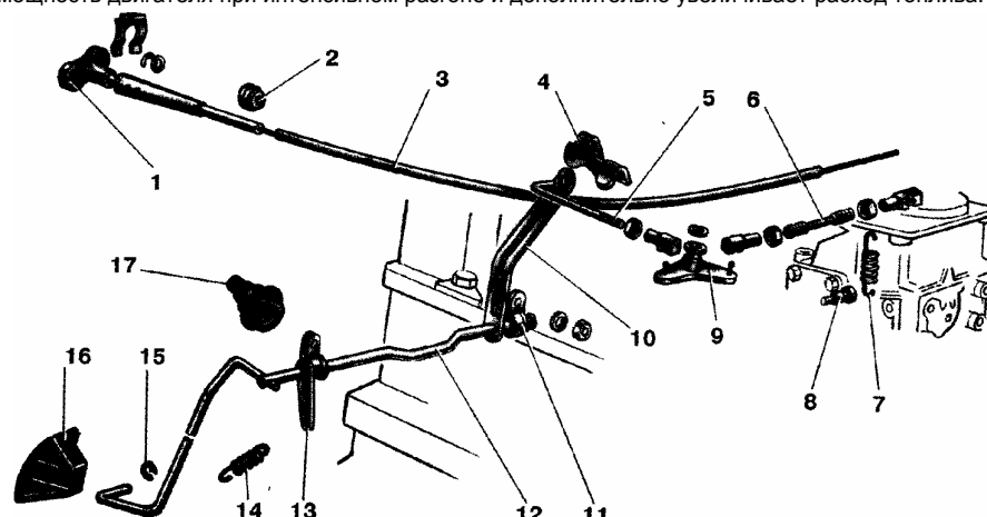
Рис. 11. Механизм управления карбюратором: 1 - рукоятка тяги управления воздушной заслонкой; 2, 17 - уплотнители; 3 - тяга управления воздушной заслонкой; 4 - скоба крепления продольной тяги; 5 - продольная тяга; 6 - поперечная тяга; 7, 14 - возвратные пружины; 8 - винт крепления возвратной пружины; 9 - промежуточный рычаг; 10, 13 - рычаги; 11 - кронштейн крепления валика; 12 - валик; 15 - стопорная шайба; 16 - педаль управления дроссельными заслонками
