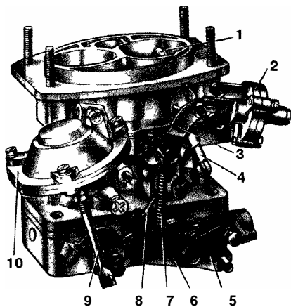
Рис. 12. Вид на карбюратор со стороны привода дроссельных заслонок: 1 - воздушная заслонка, 2 - пусковое устройство, 3 - рычаг управления воздушной заслонкой, 4 - телескопическая тяга, 5 - рычаг привода дроссельной заслонки первичной камеры, 6 - рычаг, ограничивающий открытие дроссельной заслонки вторичной камеры, 7 - возвратная пружина, 8 - тяга, связывающая дроссельную заслонку первичной камеры с рычагом управления воздушной заслонкой, 9 - шток пневмопривода 10 - пневмопривод
