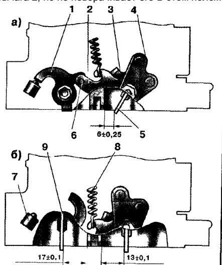
Рис. 22. Схема регулировки положения дроссельных заслонок: а - частичное открытие дроссельной заслонки первичной камеры, б - полное открытие дроссельных заслонок, 1 - рычаг на оси дроссельной заслонки 2 - рычаг ограничивающий открытие дроссельной заслонки вторичной камеры, 3 - рычаг жестко связанный с осью дроссельных заслонок, 4 - рычаг привода, 5 - дроссельная заслонка первичной камеры 6 - штифт, 7 - упор 8 - пружина 9 - дроссельная заслонка вторичной камеры
