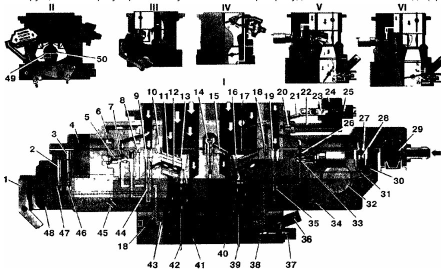
Рис. 16. Схема работы карбюратора ДАА3-2105:1 - 1 - схема работы карбюратора на максимальной мощности, II - схема работы пневмопривода дроссельной заслонки вторичной камеры, III - схема работы ускорительного насоса, IV - схема работы пускового устройства, V - схема работы карбюратора на режимах дросселирования, VI - схема работы карбюратора на холостом ходу, 1 - рычаг ускорительного насоса, 2 - винт регулировки подачи топлива ускорительным насосом, 3 - пробка обратного клапана ускорительного насоса, 4 - поплавковая камера, 5 - топливный жиклер переходной системы вторичной камеры, 6 - воздушный жиклер эконостата, 7 - воздушный жиклер переходной системы, 8 - топливный жиклер переходной системы, 9 - главный воздушный жиклер вторичной камеры, 10 - эмульсионный жиклер эконостата, 11 - распылитель эконостата, 12 - распылитель главной дозирующей системы вторичной камеры, 13 - малый диффузор вторичной камеры, 14 - клапан распылителя ускорительного насоса, 15 - распылитель ускорительного насоса, 16 - малый диффузор первичной камеры, 17 - воздушная заслонка, 18 - соединительные втулки каналов карбюратора, 19 - главный воздушный жиклер первичной камеры, 20 - воздушный жиклер пускового устройства, 21 - тяга, соединяющая рычаг оси воздушной заслонки с рейкой пускового устройства, 22 - корпус пускового устройства, 23 - рейка пускового устройства, 24 - диафрагма пускового устройства, 25 - регулировочный винт пускового устройства, 26 - воздушный жиклер системы холостого хода, 27 - седло игльчатого клапана, 28 - игльчатый клапан, 29 - топливный фильтр, 30 - кронштейн поплавка с упором и язычком, 31 - демпфирующий шарик, 32 - поплавок, 33 - топливный жиклер системы холостого хода, 34 - главный топливный жиклер первичной камеры, 35 - эмульсионная трубка первичной камеры, 36 - регулировочный винт качества смеси системы холостого хода, 37 - регулировочный винт количества смеси системы холостого хода, 38 - седло регулировочного винта, 39 - дроссельная заслонка первичной камеры, 40 - первичная смесительная камера, 41 - вторичная смесительная камера, 42 - дроссельная заслонка вторичной камеры, 43 - нерегулируемые отверстия переходной системы, 44 - эмульсионная трубка вторичной камеры, 45 - главный топливный жиклер вторичной камеры, 46 - обратный клапан, 47 - перепускной жиклер ускорительного насоса, 48 - диафрагма ускорительного насоса, 49 - жиклер пневмопривода, расположенный во вторичной камере 50 - жиклер пневмопривода, расположенный в первичной камере
