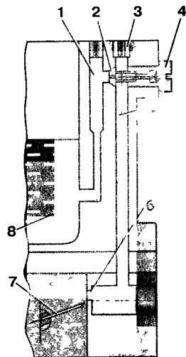
Рис. 8. Переходная система вторичной камеры: 1 - топливный канал; 2 - топливный жиклер; 3 - воздушный жиклер; 4 - корпус жиклера; 5 - эмульсионный канал; 6 - выходные отверстия; 7 - дроссельная заслонка; 8 - поплавковая камера
