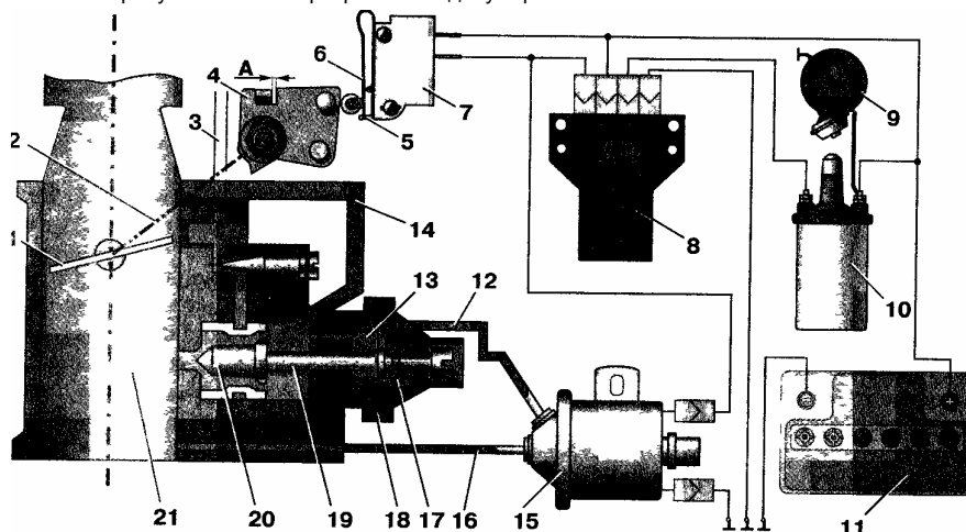
Рис. 9. Схема системы ЭПХХ: 1 - дроссельная заслонка; 2 - рычаг; 3 - эмульсионный канал; 4 - рычаг привода; 5 - ограничитель; 6 - пружина; 7 - микропереключатель; 8 - блок управления; 9 - прерыватель-распределитель; 10 - катушка зажигания; 11 - аккумуляторная батарея; 12 - канал; 13 - наддиафрагменная полость; 14 - обводной канал; 15 - электропневматический клапан; 16 - соединительный канал; 17 - поддиафрагменная полость; 18 - диафрагма; 19 - шток; 20 - игла; 21 - задрроссельное пространство
