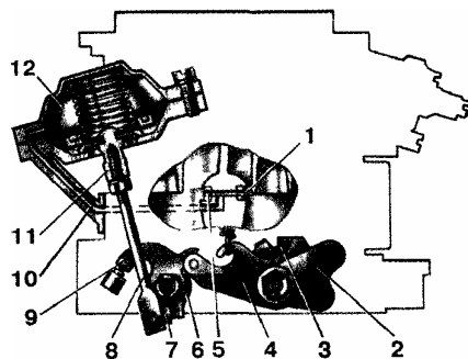
Рис. 13. Привод дроссельной заслонки вторичной камеры карбюраторов ДААЗ-2105 и -2107: 1 - жиклер пневмопривода, расположенный в диффузоре первичной камеры, 2 - рычаг привода дроссельных заслонок, 3 - рычаг, жестко связанный с осью дроссельной заслонки, 4 - блокирующий рычаг, 5 - жиклер пневмопривода, расположенный в диффузоре вторичной камеры, 6 - промежуточный рычаг, 7 - пружина дроссельной заслонки вторичной камеры, 8 - шток пневмопривода, 9 - рычаг управления дроссельной заслонкой вторичной камеры, 10 - канал подвода разрежения в пневмопривод, 11 - втулка штока, 12 - рабочая полость пневмопривода дроссельной заслонки вторичной камеры
