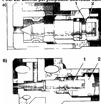
Рис. 26. Винты количества (а) и качества (б) смеси системы холостого хода карбюратора «Озон» без ЭПХХ: 1 - регулировочный винт, 2 - ограничительная втулка
