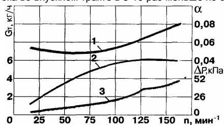
Рис. 3. Скоростная пусковая характеристика карбюратора малолитражного двигателя: 1 - состав горючей смеси, 2 - расход топлива; 3 - разрежение во ВТ
