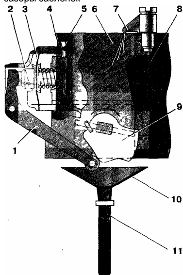
Рис. 24. Схема проверки подачи ускорительного насоса: 1 - рычаг привода, 2 - толкатель, 3 - диафрагма, 4 - обратный клапан, 5 - ограничитель хода клапана, 6 - главный воздушный канал, 7 - распылитель, 8 - канал, 9 - кулачок, 10 - воронка, 11 - мерная мензурка
