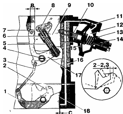
Рис. 4. Пусковое устройство: 1 - рычаг; 2 - выступ 3, 9 - тяги, 4 - винт, 5 - телескопическая тяга, 6, 10 - штоки, 7 - воздушная заслонка, 8 - рычаг, 11 - диафрагма, 12 - наддиафрагменная полость, 13-пружина, 14 - регулировочный винт, 15 - поддиафрагменная полость, 16-канал, 17 - трехплечий рычаг, 18 - дроссельная заслонка
