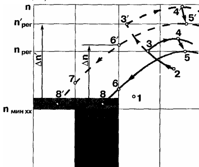
О 1,5 3 4,5 CO, % Рис. 29. Схема регулировки СХХ
