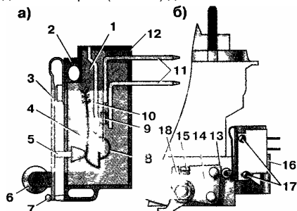
Рис. 30. Устройство микропереключателя и его расположение на карбюраторе: а - устройство микропереключателя; б - размещение микропереключателя; 1 - полость корпуса; 2 - микропереключатель; 3 - пластинчатый рычаг; 4 - плоская пружина; 5 - толкатель; 6 - ролик; 7 - ограничитель перемещения рычага 3; 8 - перебрасывающая пружина; 9 - подвижные контакты; 10 - ограничитель перемещения контактов; 11 - электрические выводы; 12 - корпус; 13 - контактирующая поверхность; 14 - рычаг привода дроссельной заслонки первичной камеры; 15 - усик рычага; 16 - кронштейн; 17 - винты крепления; 18 - ось дроссельной заслонки
