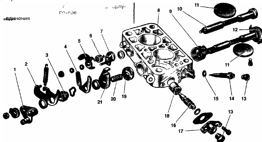
Рис. 19. Детали корпуса дроссельных заслонок: 1 - рычаг привода дроссельных заслонок, 2 - рычаг, ограничивающий открытие дроссельной заслонки вторичной камеры, 3 - втулка, 4 - рычаг связи с воздушной заслонкой, 5 - рычаг, закрепленный на оси дроссельной заслонки вторичной камеры, 6 - пружина, 7 - рычаг, связанный с пневмоприводом, 8 - корпус дроссельных заслонок, 9 - возвратная пружина дроссельной заслонки первичной камеры, 10 - ось дроссельной заслонки вторичной камеры, 11 - дроссельные заслонки, 12 - ось дроссельной заслонки первичной камеры, 13 - ограничительные втулки, 14 - винт регулировки качества смеси системы холостого хода, 15 - уплотнительное кольцо, 16 - винт регулировки количества смеси, 17 - втулка винта количества смеси, 18 - смесительная втулка, 19 - золотник, 20 - пружина золотника, 21 - рычаг оси дроссельной заслонки первичной камеры
