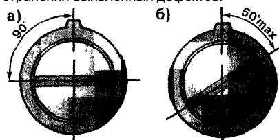
Рис. 27. Установка ограничительных втулок на винты регулировки СХХ: а - винт количества смеси, б - винт качества смеси
