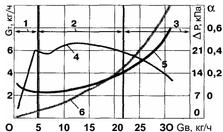
Рис. 2. Пусковая характеристика карбюратора малолитражного двигателя: 1, 2 и 3 - участки характеристики, 4 - расход топлива; 5 - состав горючей смеси, 6 - разрежение во ВТ
