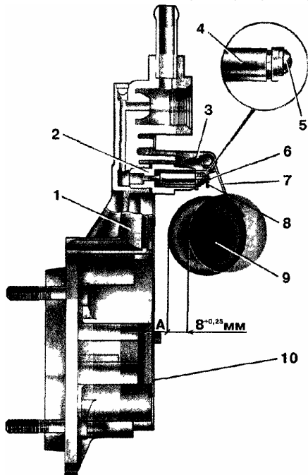
Рис. 21. Схема установки уровня топлива в поплавковой камере: 1 - крышка карбюратора; 2 - седло игольчатого клапана, 3 - упор, 4 - игольчатый клапан; 5 - шарик игольчатого клапана; 6 - оттяжная вилка игольчатого клапана, 7 - кронштейн поплавка, 8 - язычок; 9 - поплавок, 10 - прокладка
